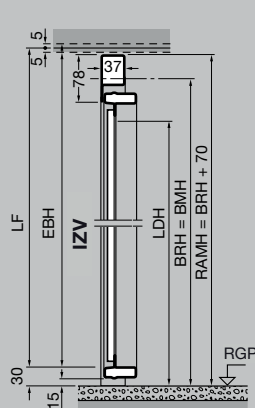
Vertikalni presjek vrata bez donjeg nosača
