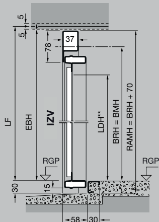
Vertikalni presjek vrata s donjim nosačem
