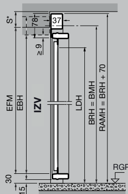
Vertikalni presjek vrata bez donjeg nosača
