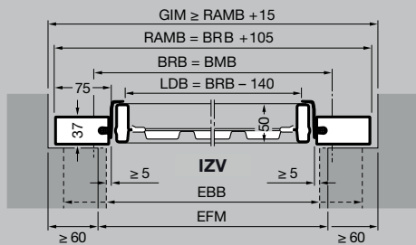
Vertikalni presjek vrata s donjim nosačem
